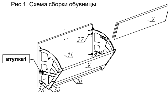
Рис.1. Схема сборки обувницы
