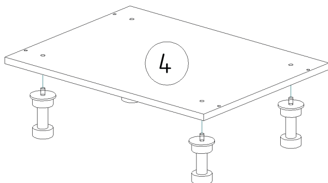
Рис. 2 Установка опор+клипса+планка (установка опор на саморезы 4x16 мм и винта к опоре, установка планки на саморезы 4x16 мм)
